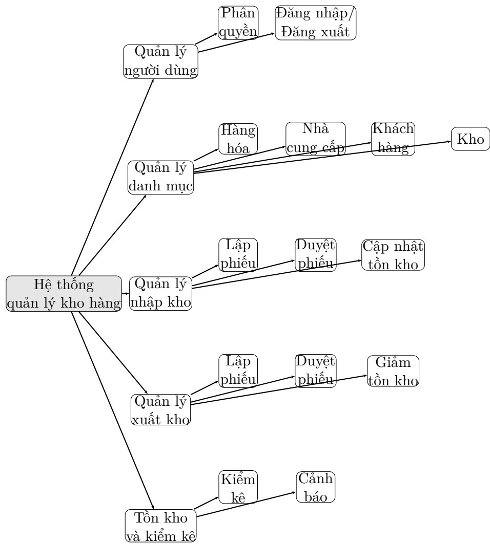
Figure 1: Sơ đồ phân cấp chức năng (BFD) hệ thống quản lý kho hàng
